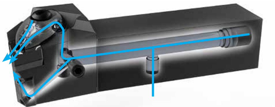
JETI - interne Kühlschmierstoffzufuhr mit strömungsoptimierter Pratze
